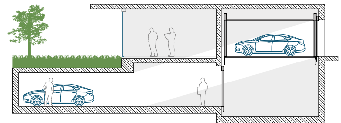
Grijs vlak = Vereiste ruimte voor een conventionele hellingbaan
